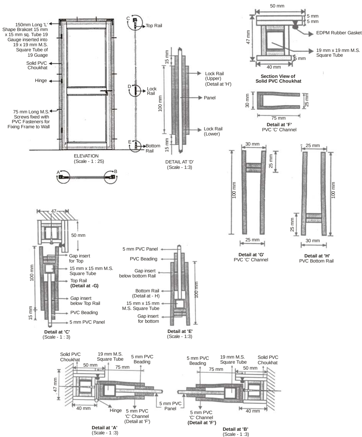
Fig. 9.21 : PVC Door Frame
