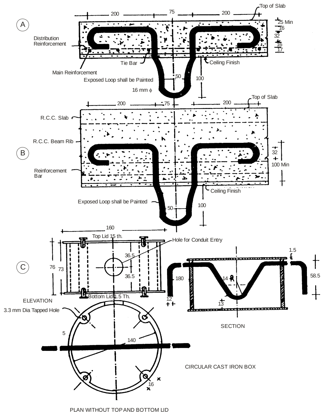
Fig. 10.9 : Fan Clamps
